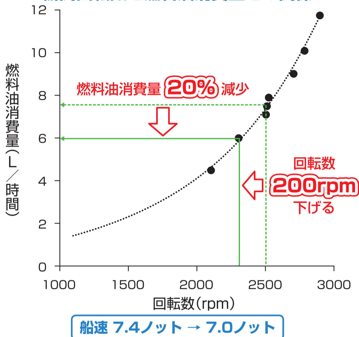
機関回転数と燃料油消費量との関係
