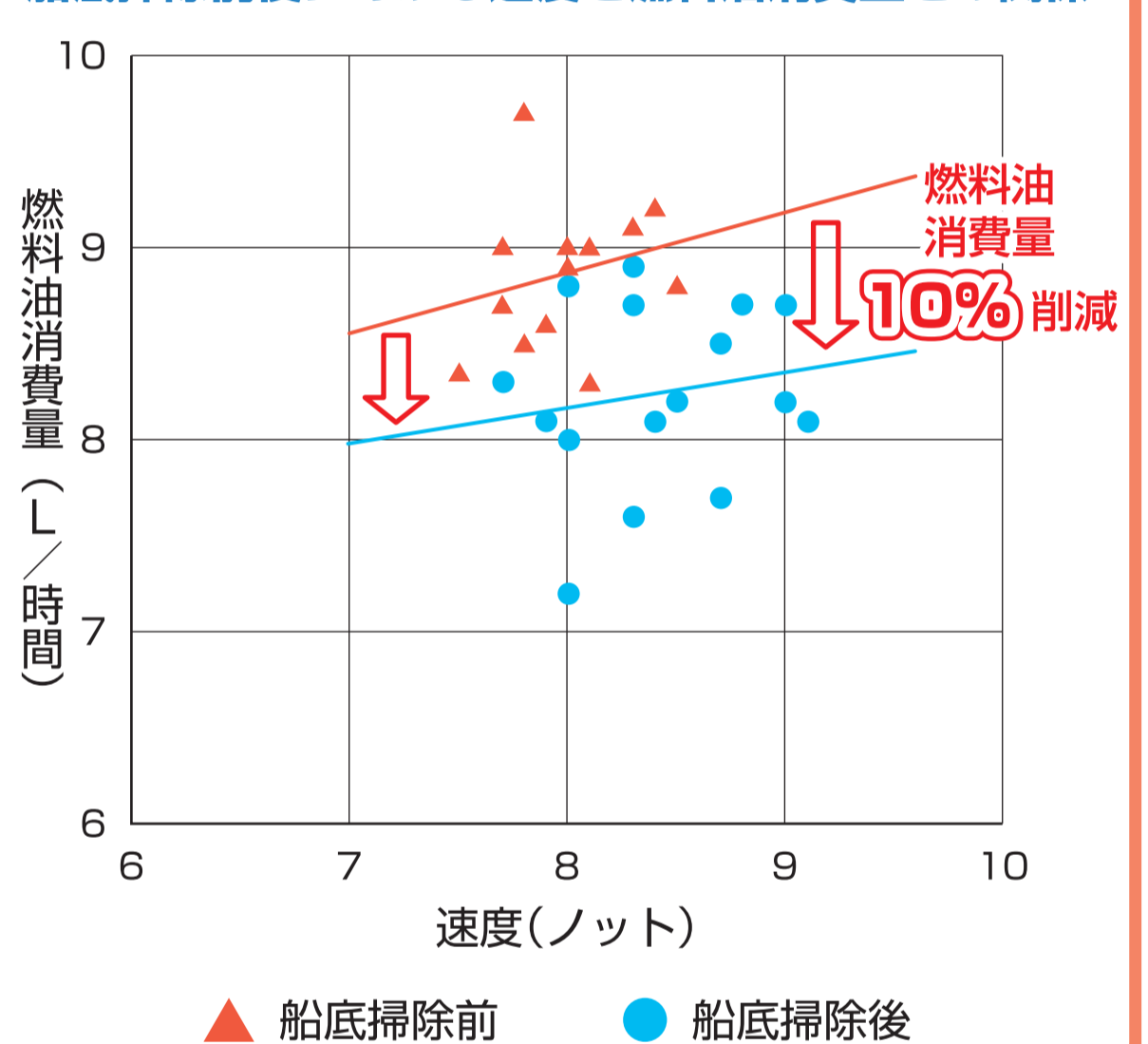
船底掃除前後における速度と燃料油消費量との関係
